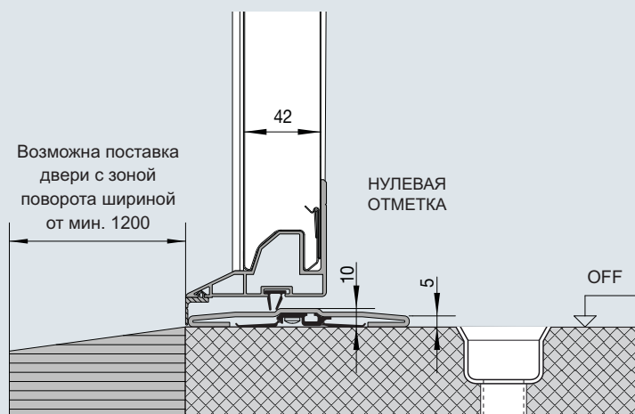
Отдельно устанавливаемые уплотнители для ворот с калиткой сглаживают неровности пола.
