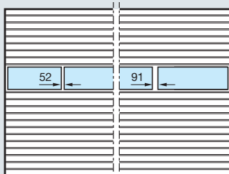
С алюминиевыми рамами остекления. Высота рамы: 500, 625, 750 мм. Вариант N с узкими и вариант B с широкими перекладинами.
