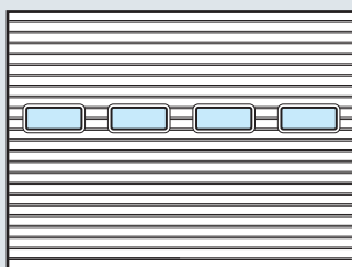
С сэндвичными окнами, тип A Размер проема в свету: 635 x 245 мм Для секций ворот высотой 500, 625, 750 мм
