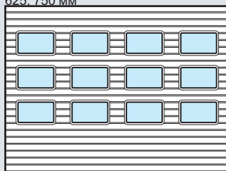
С сэндвичными окнами, тип E Размер проема в свету: 725 x 370 мм Для секций ворот высотой 625, 750 мм
