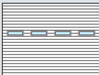
С сэндвичными окнами, тип D Размер проема в свету: 602 x 132 мм Для секций ворот высотой 500, 625, 750 мм
